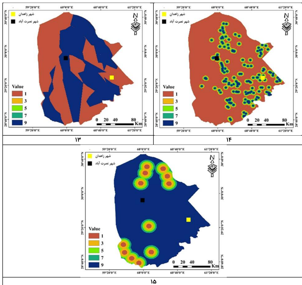
شکل ۲. نقشه‌های استانداردسازی شده (۱. ارتفاع، ۲. شیب، ۳. جهت شیب، ۴. فاصله از آبراهه، ۵. فاصله از دشت سیلابی، ۶. فاصله از گسل، ۷. خاک، ۸. زمین‌شناسی، ۹. کاربری اراضی، ۱۰. دما، ۱۱. بارش، ۱۲. فاصله از آبراهه، ۱۳. وضعیت توپوگرافی (دشت و کوهستان)، ۱۴. فاصله از مراکز سکونتگاهی، ۱۵. فاصله از مخروط‌افکنه).
