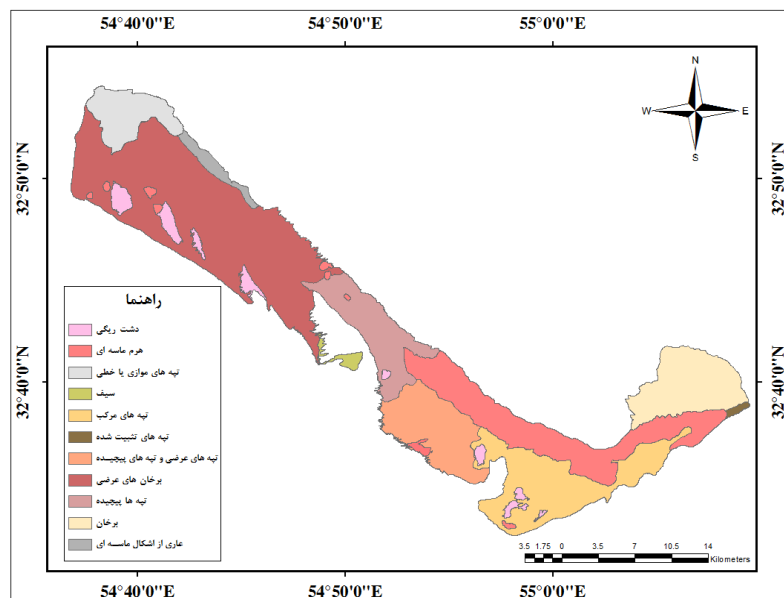
شکل ۵- نقشه پراکنش مکانی مورفولوژی تپه‌های ماسه‌ای ریگ زیرین
