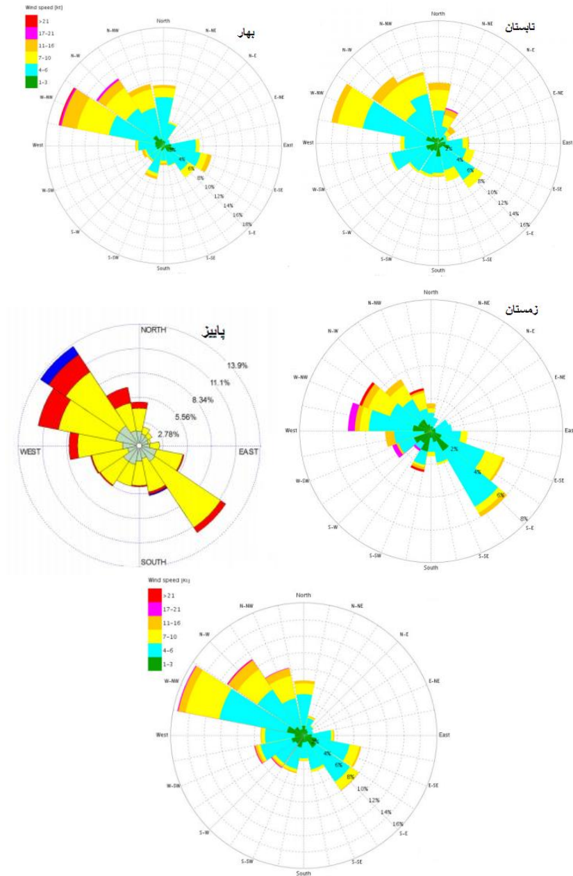
شکل ۸- گلبادهای فصلی و سالانه ایستگاه سینوپتیکی یزد (برگرفته از سایت هواشناسی استان یزد)
