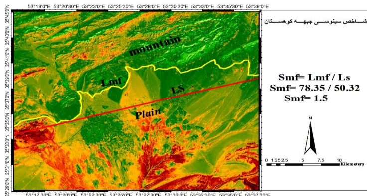
شکل ۷- ارزیابی شاخص Smf برای حوضه سمنان
