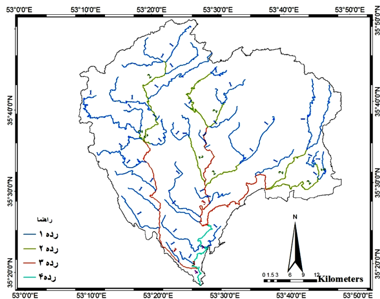
شکل ۵. رده بندی به روش استرالر حوضه سمنان
