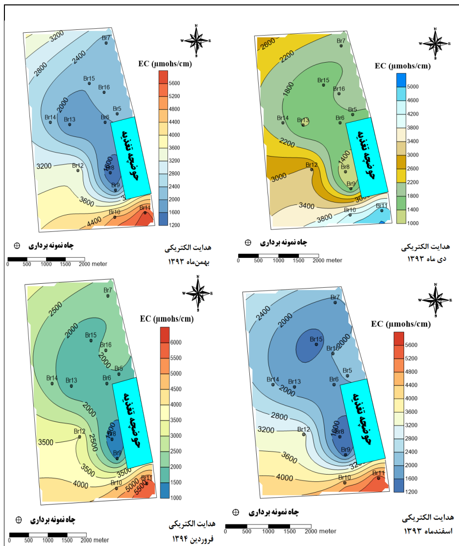
شکل ۵- تغییرات مکانی هدایت الکتریکی آب زیرزمینی در اطراف حوضچه تغذیه آردو
