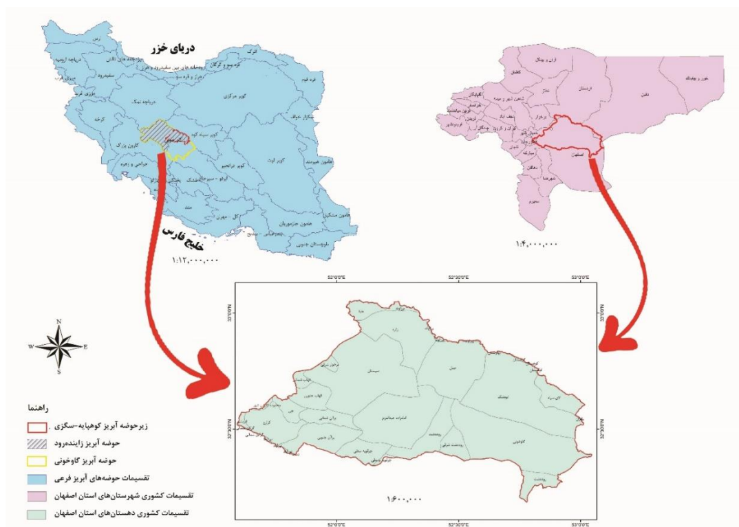
شکل ۱. موقعیت جغرافیایی زیرحوضه آبریز کوهپایه-سگزی
