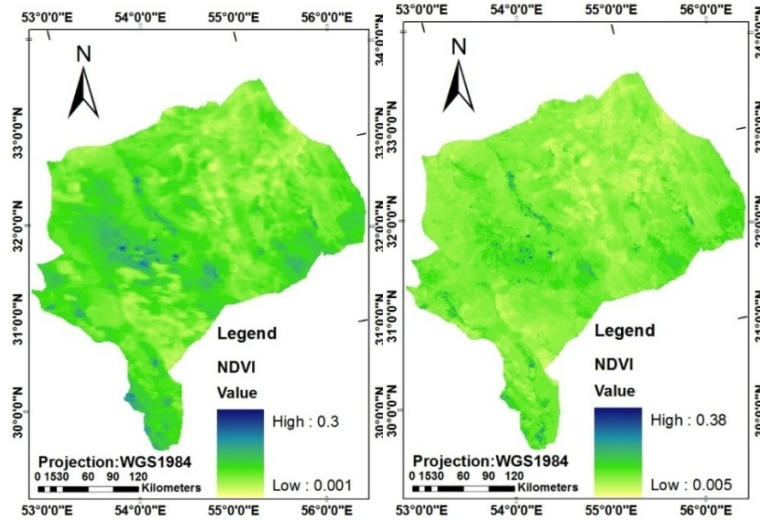
شکل ۴. نقشه NDVI مربوط به اکتبر
