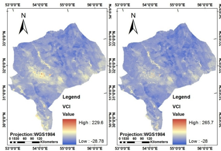
شکل ۶. نقشه VCI مربوط به اکتبر
