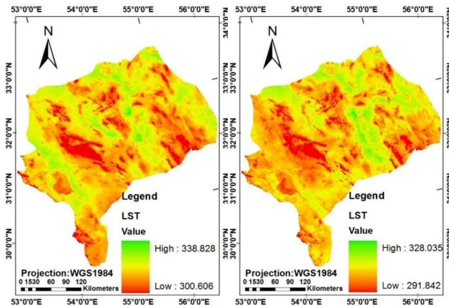
شکل ۸. نقشه LST مربوط به اکتبر
