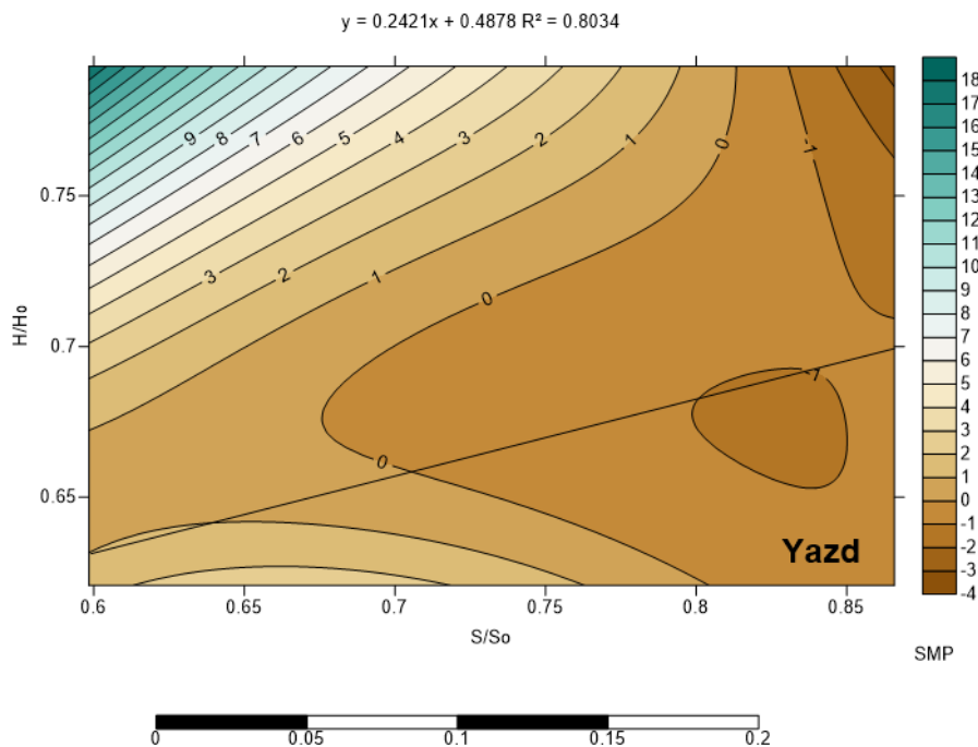
شکل ۵. نمودار TGM در ایستگاه یزد
