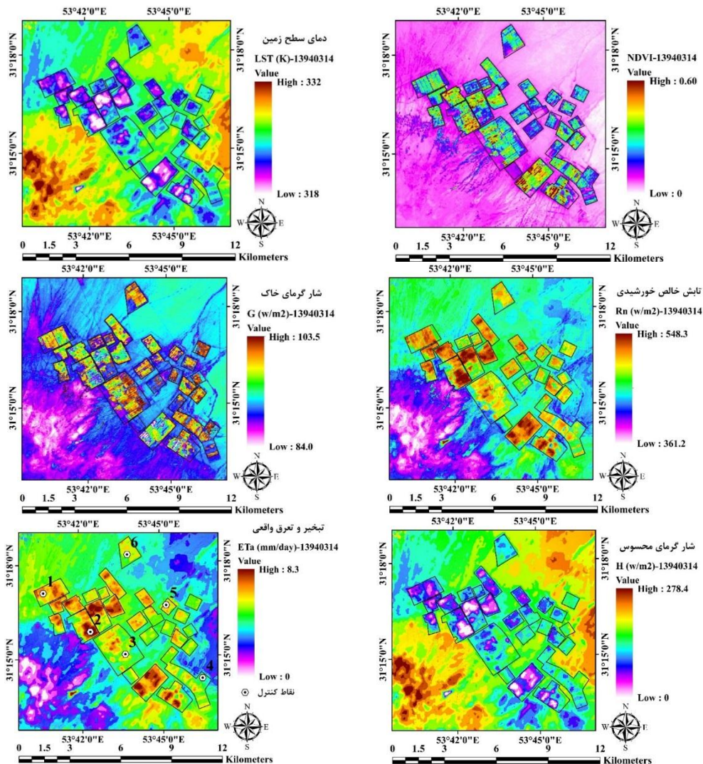
شکل ۳- یک نمونه تصویر NDVI، دمای سطح زمین، تابش خالص خورشیدی، شار گرمای خاک، شار گرمای محسوس و تبخیر و تعرق واقعی روزانه در تاریخ ۱۳۹۴/۰۳/۱۴
