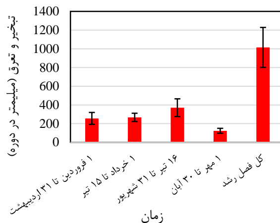
شکل ۹ - مجموع تبخیر و تعرق واقعی سبال در چهار دوره اصلی فنولوژی پسته و کل فصل رشد
