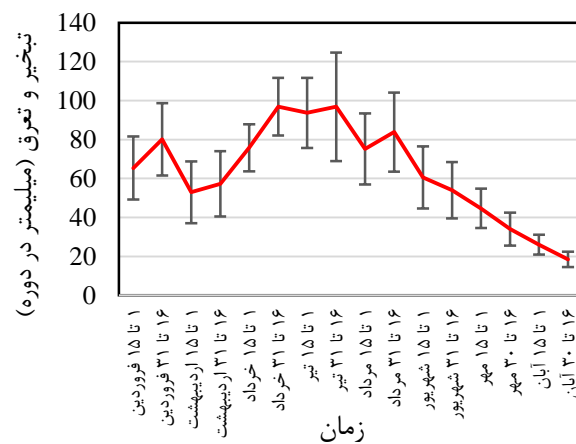
شکل ۶- میانگین میزان تبخیر و تعرق در دوره‌های ۱۵ روزه فنولوژی در سطح کل باغات پسته
